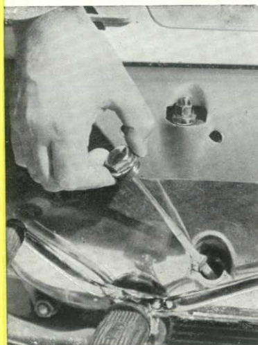
Tappo riempimento e controllo livello olio.
