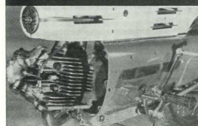
Immediata possibilità di smontaggio della candela e di registrazione delle valvole
