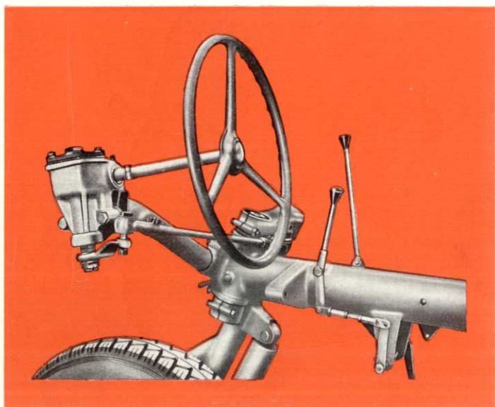
Gruppo comando sterzo
