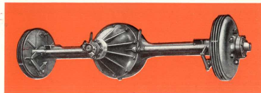
Gruppo ponte differenziale
